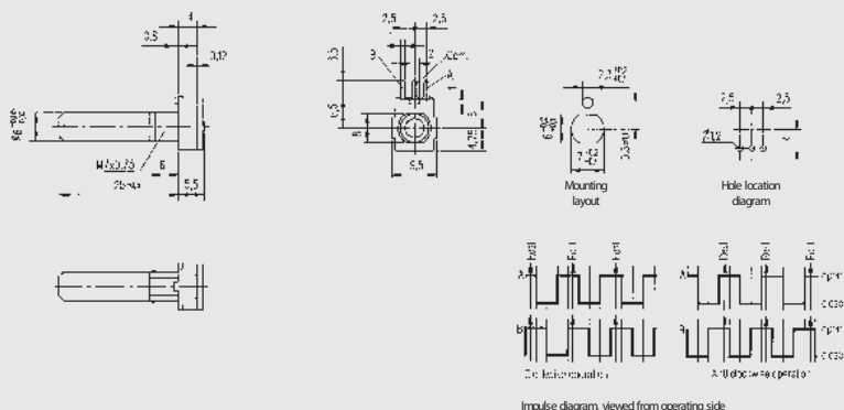
BG10 · Radial
