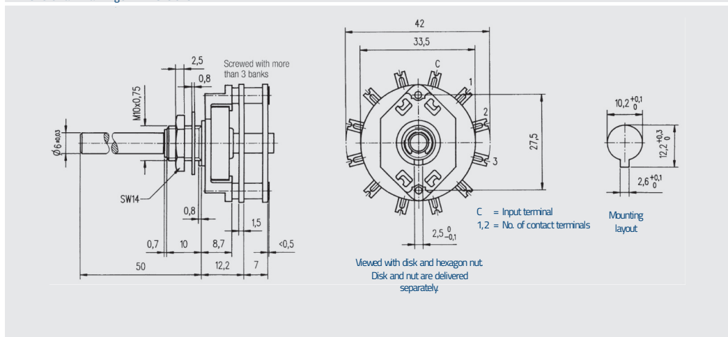
SM 30 · Standard version
