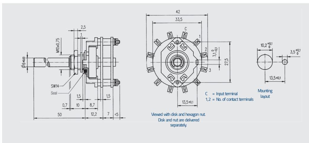
SM 30 · MIL version
