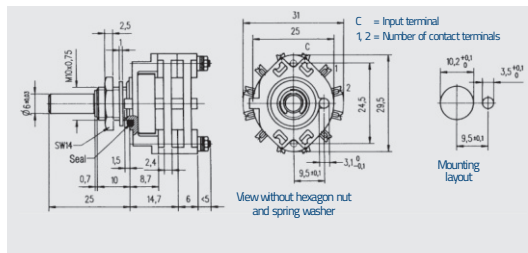
SM25 · Watertight version. Non-turn tab 9,5 mm
