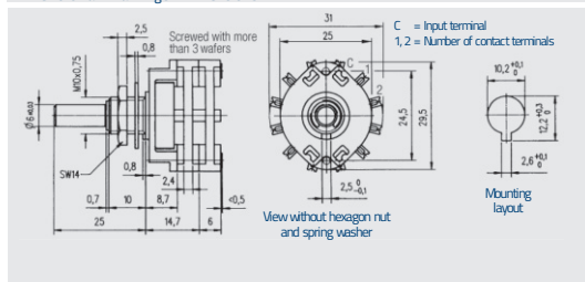
SM25 · Standard version
