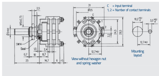
SM25 · Watertight version. Non-turn tab 12,7 mm
